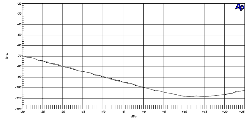
Audio Precision DMC THD+N vers AMPL Input - Rec Out 12/01/04 11:46:54
